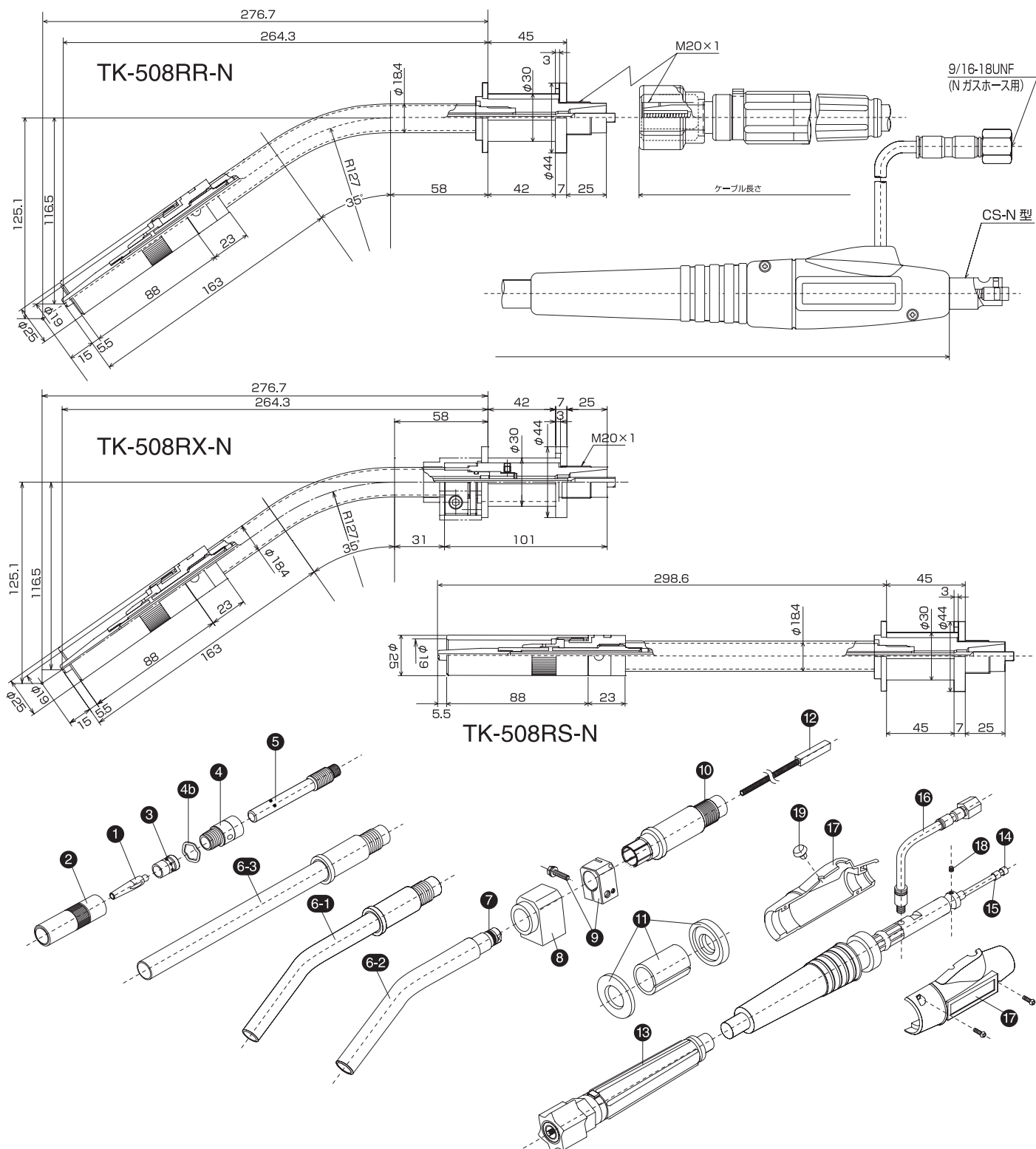
TK-508RR-N/508RX/508RS-N 部品リスト Parts List
