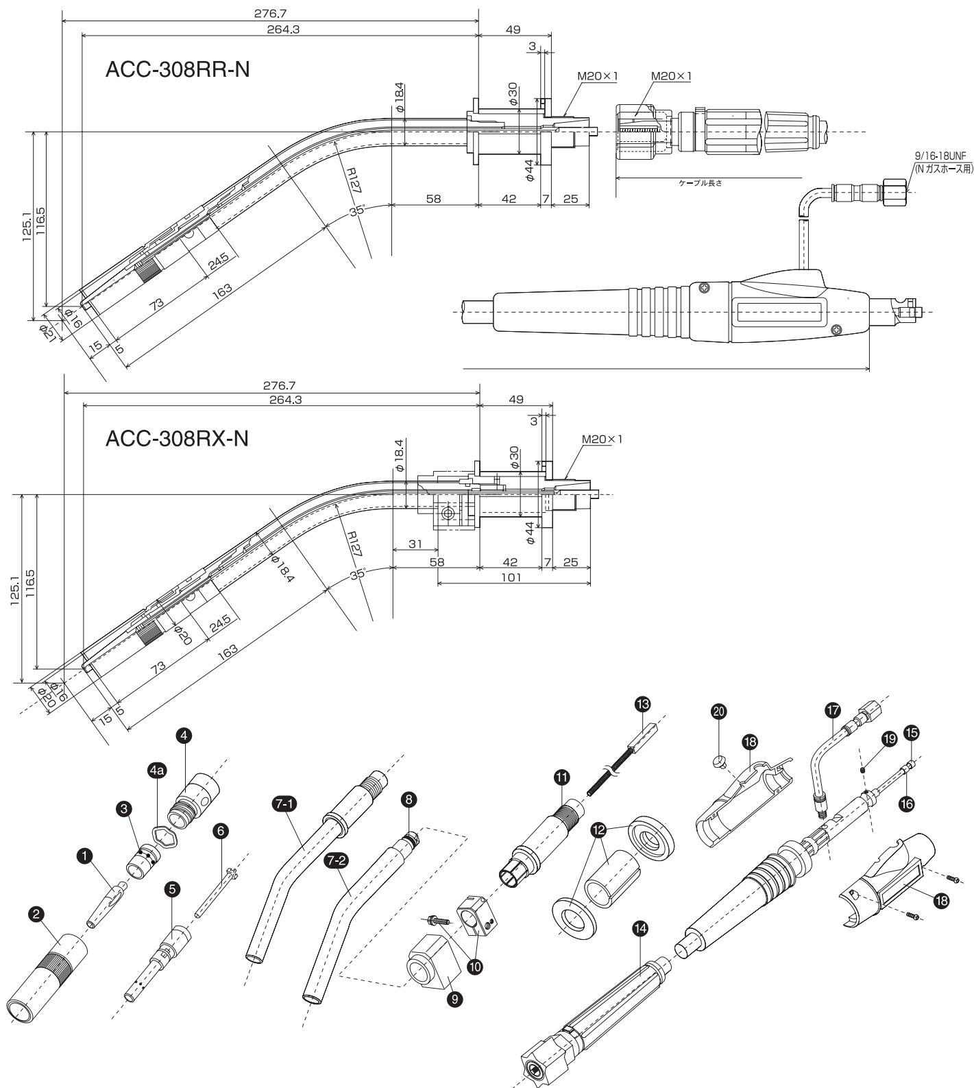
ACC-308RR-N/308RX-N 部品リスト Parts List
