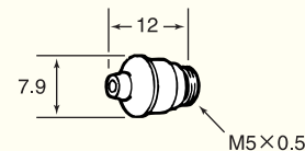
1 ノズル
