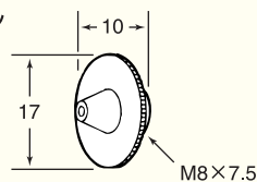
7 ノズル
