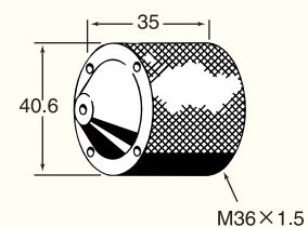
2 ノズル
