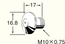
1 KOMノズル
