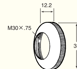
3 ナット
