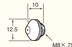
5 ノズル5" KN
