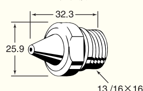
3 ノズル
