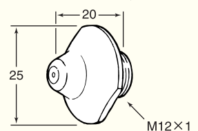
1 エコノズル
