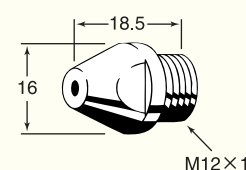
8-1 HS95ノズル
