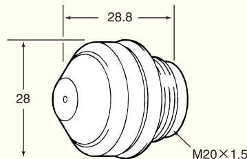
5 ノズルDL
