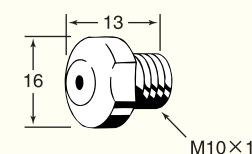
8-1 HS95ノズル
