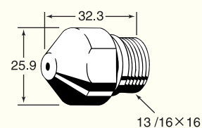
2 ノズル
