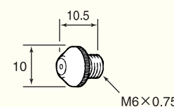
5 ノズル5" KN
